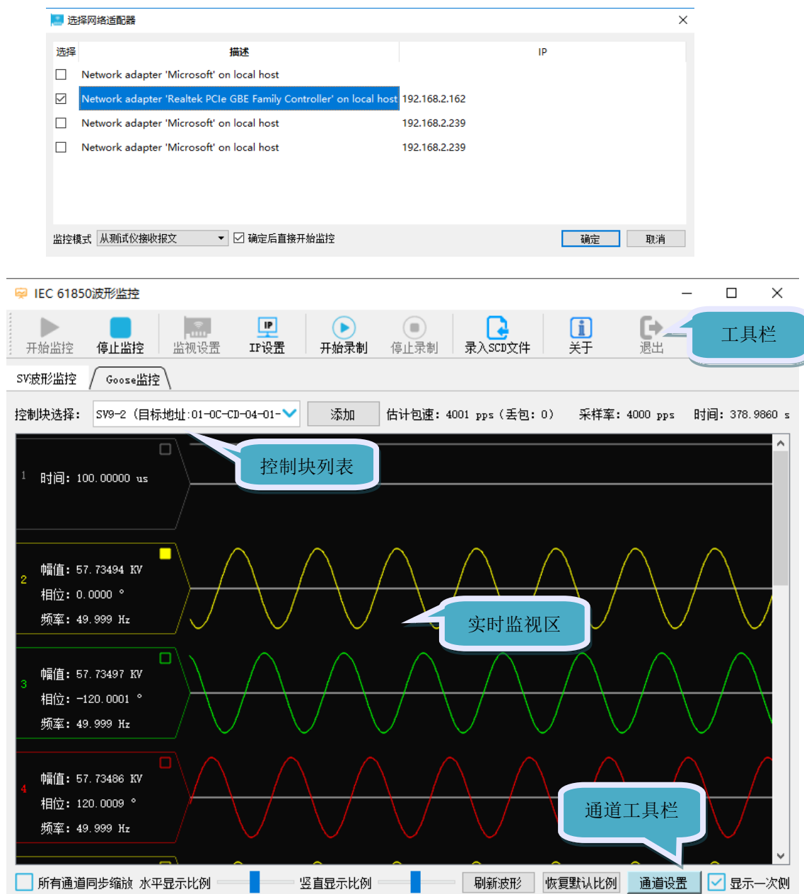
图 3-23 SV/GOOSE 报文监视
