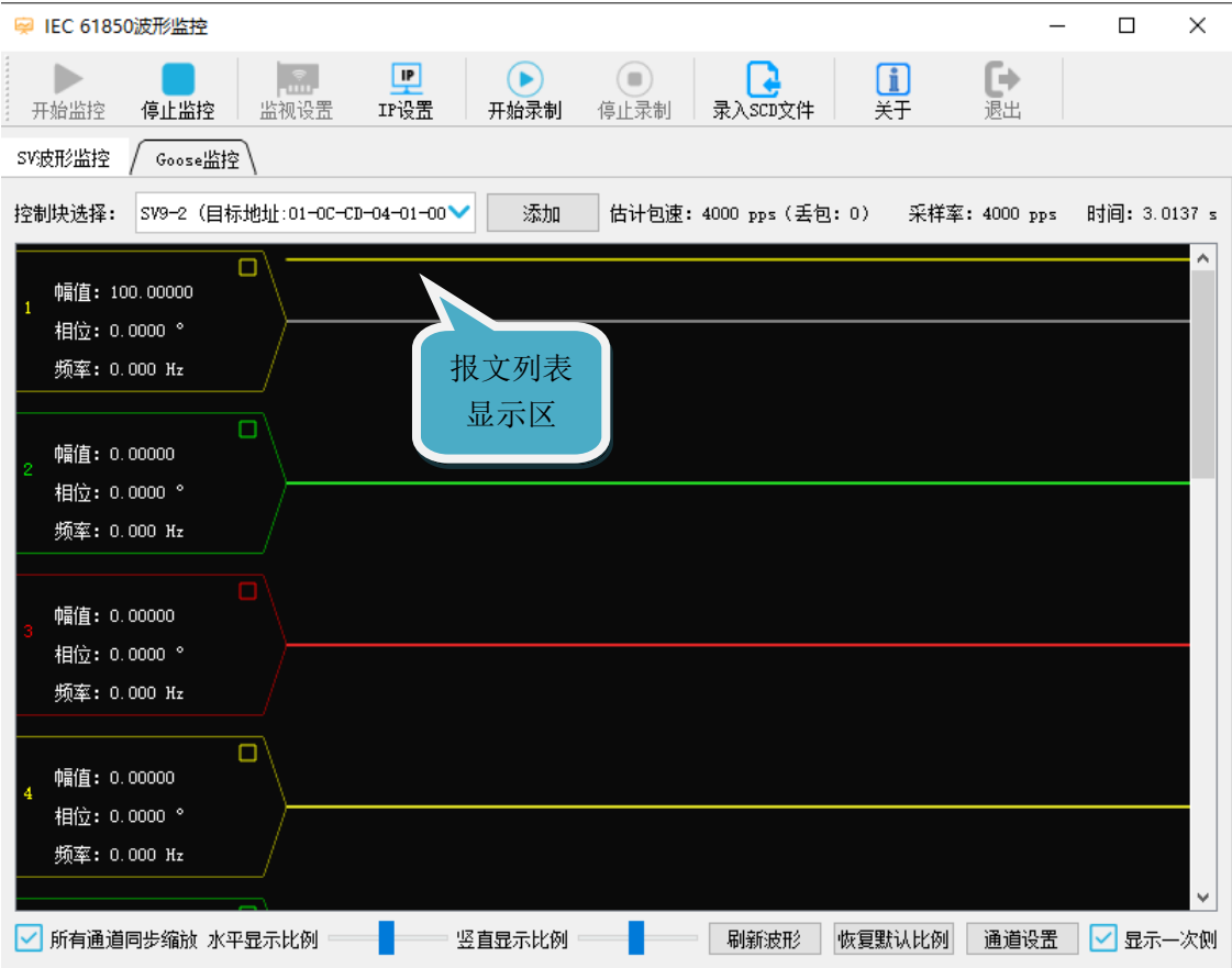
图 3-17 IEC 61850 波形监控界面
