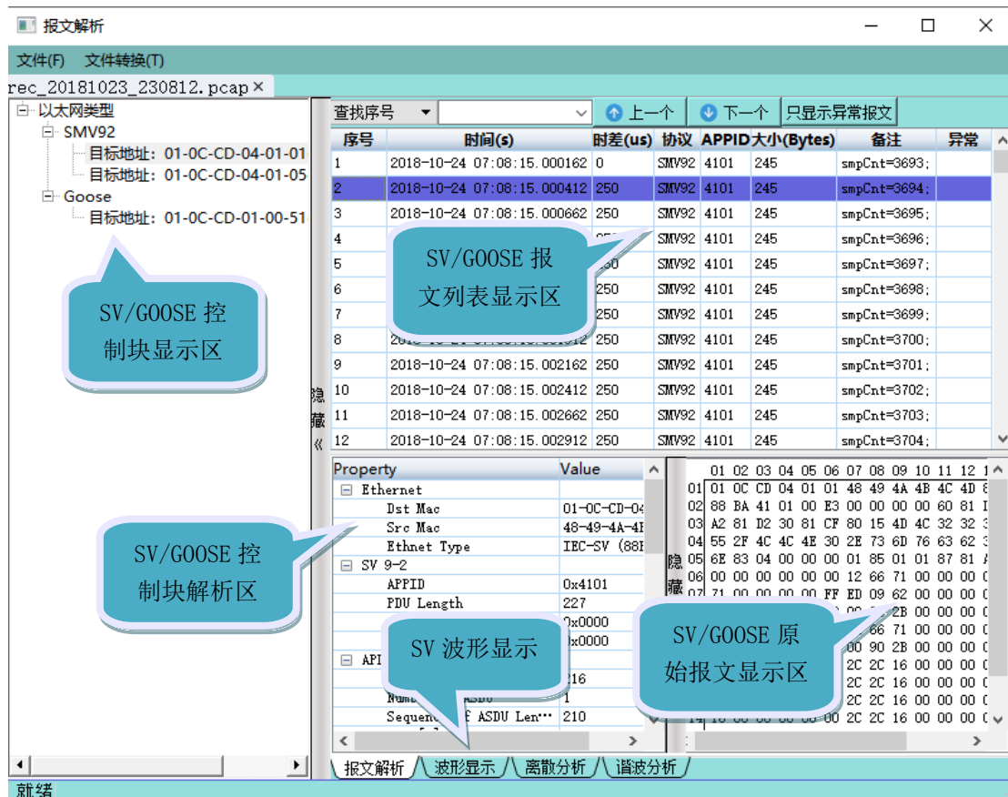
图 3-24 SV/GOOSE 报文分析
