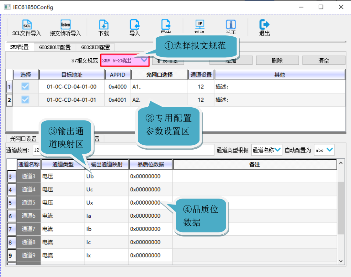
图 3-3 IEC61850-9-2 SMV 配置
