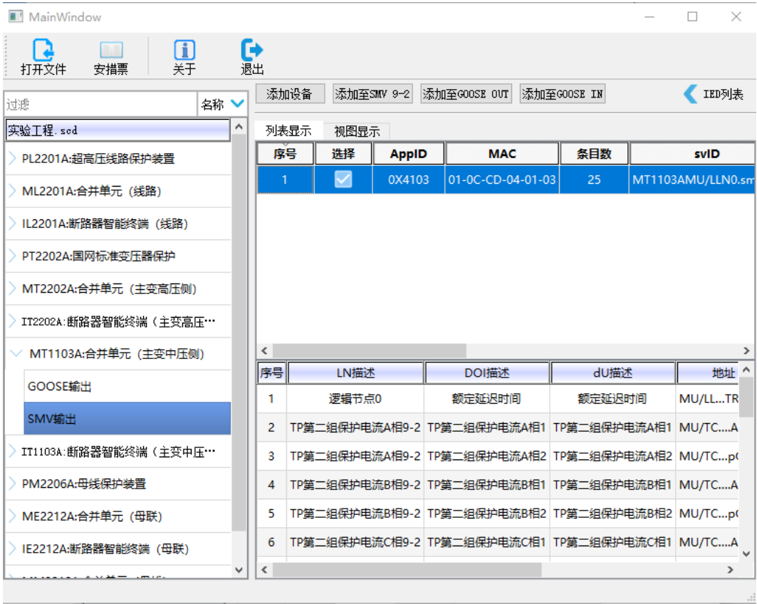
图 3-15 SCL 文件导入—导入 SMV 配置
