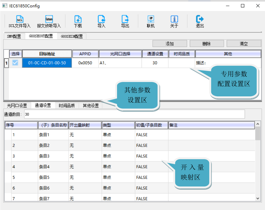
图 3-14 GOOSE OUT 配置界面
