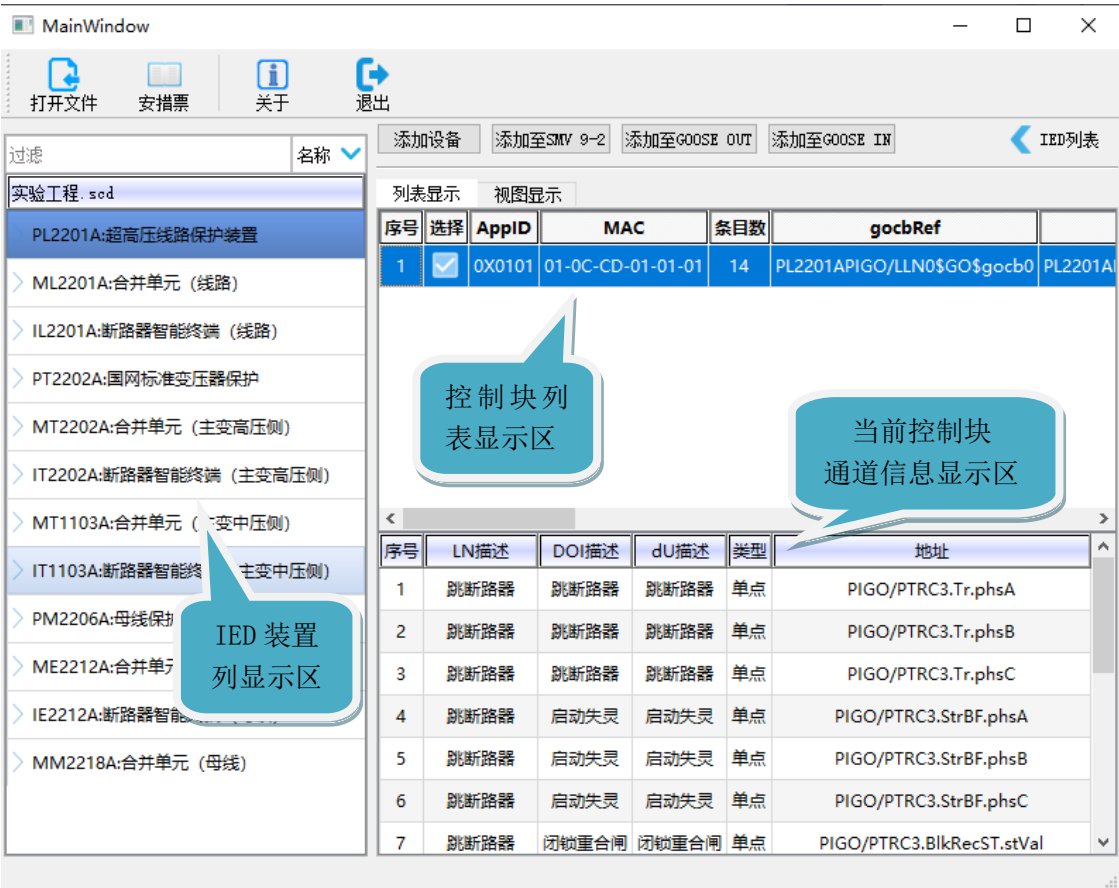
图 3-15 SCL 文件导入界面
