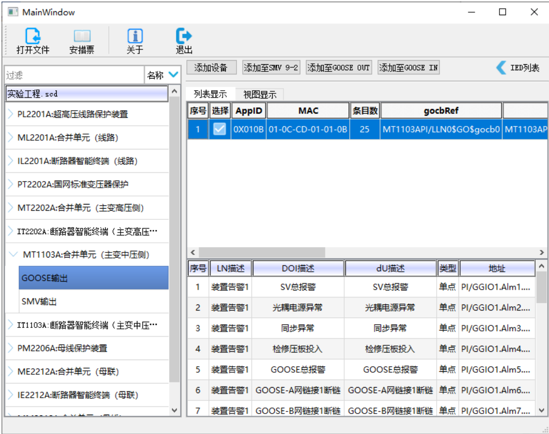
图 3-16 SCL 文件导入—导入 GOOSE 配置
