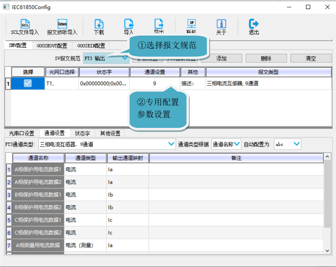
图 3-10 FT3（IEC60044-7/8）SMV 配置
